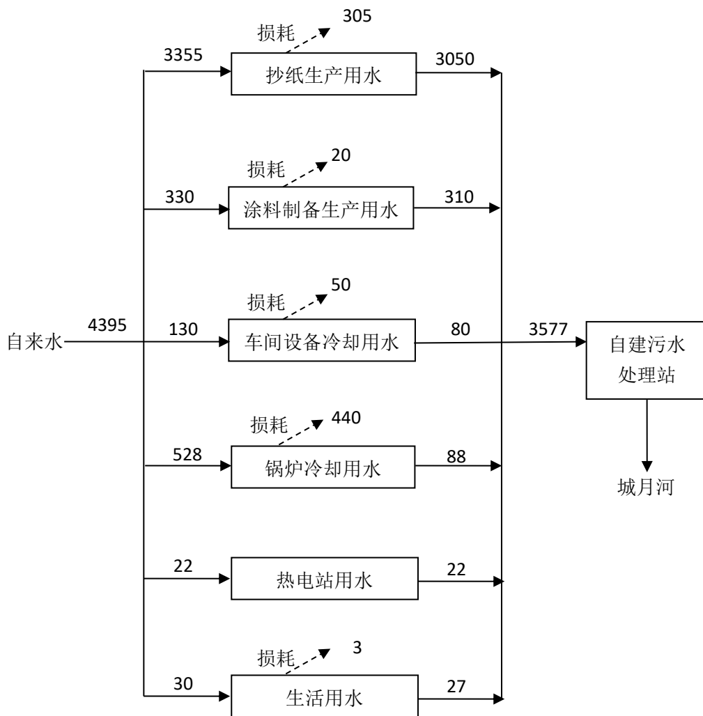
图 2.4-1 现有工程水平衡图 (单位: m³/d)
