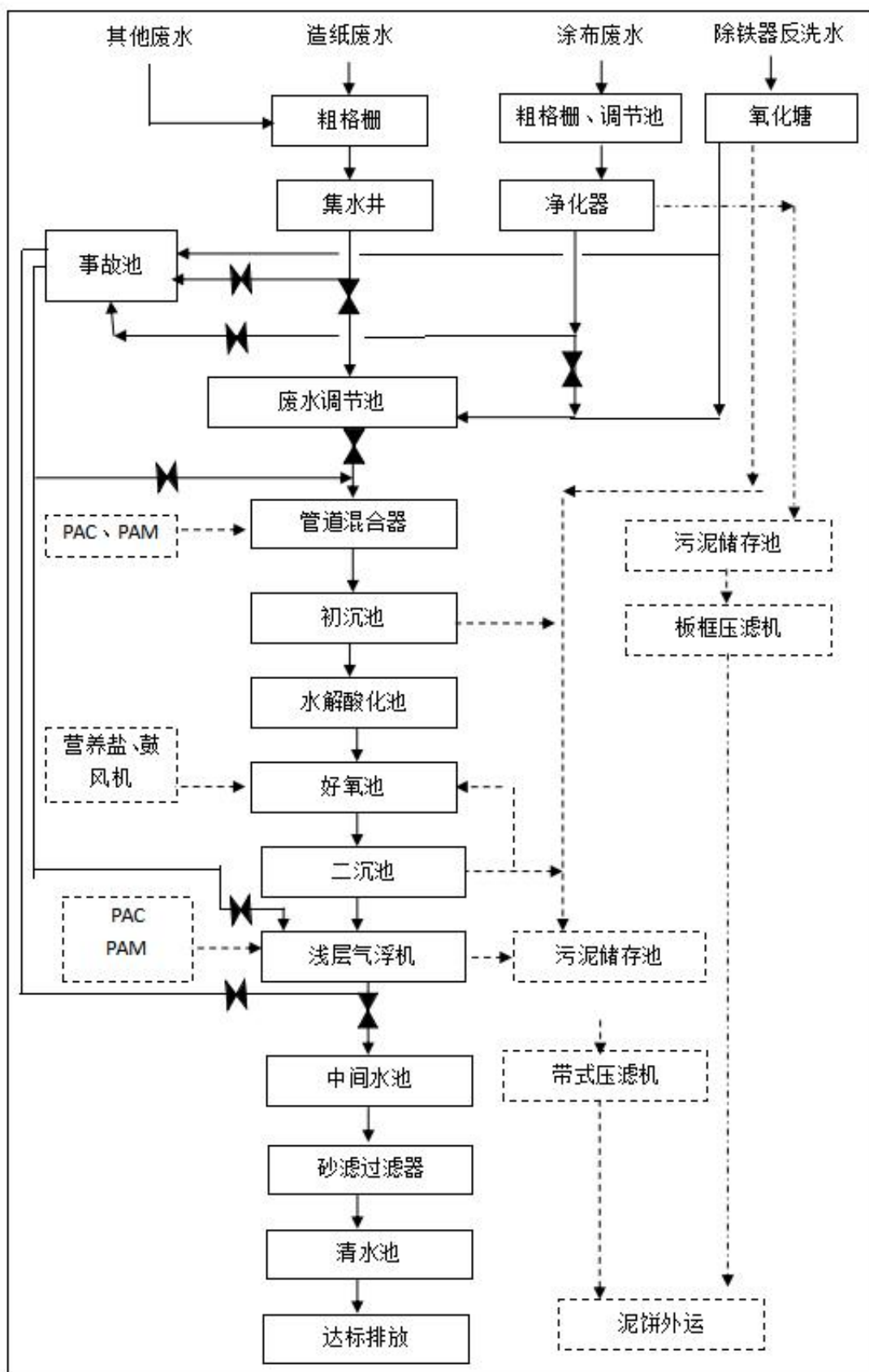
图 2.6-2 现有污水处理站处理工艺流程图
