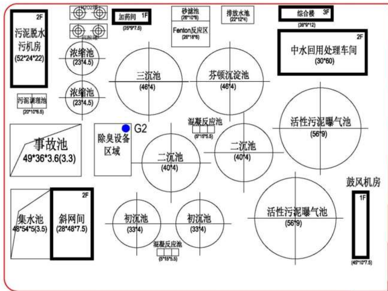
图2.2-3原地块二（污水处理系统）平面布置示意图
