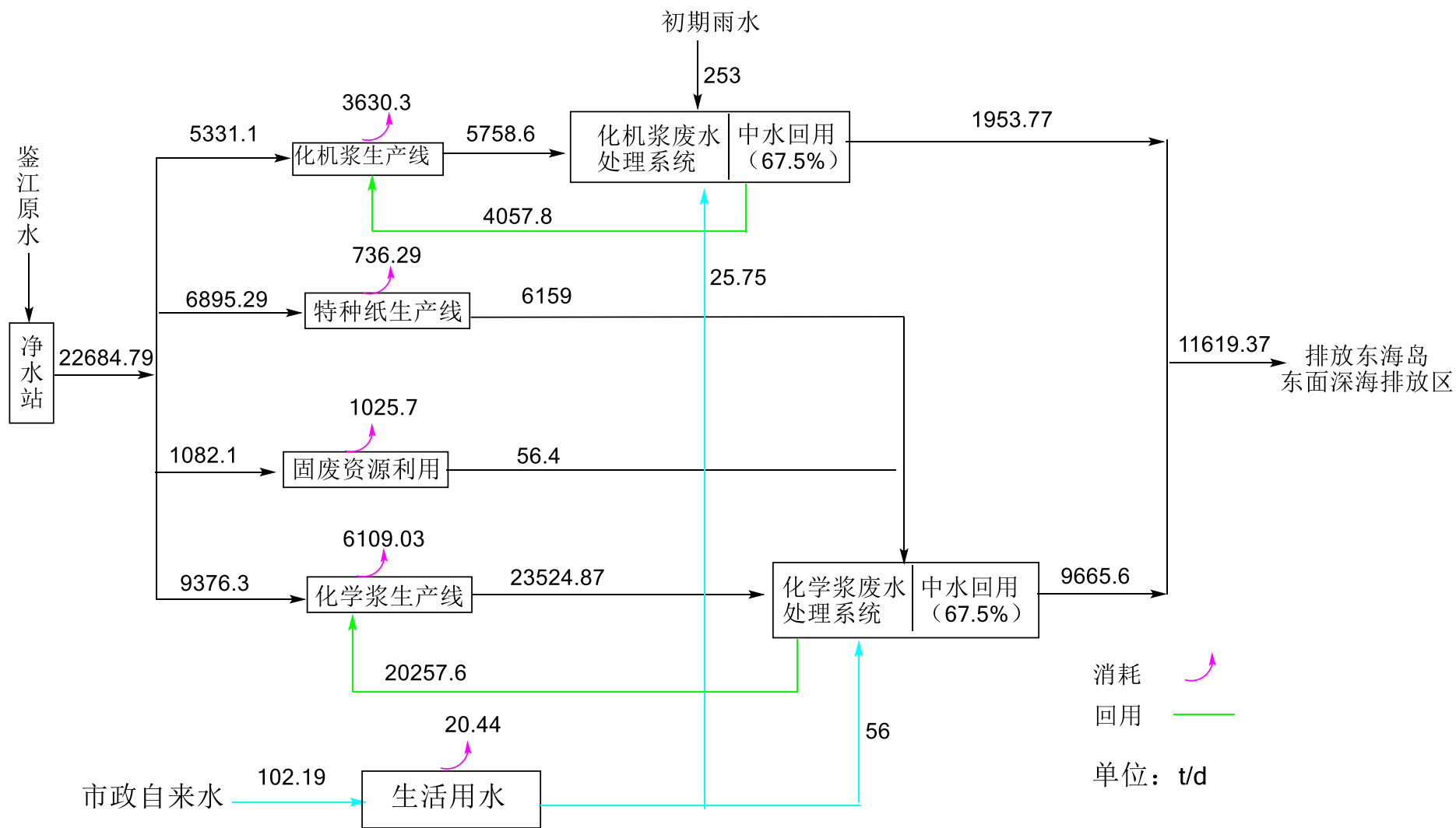
图3.2-25全厂水平衡图
