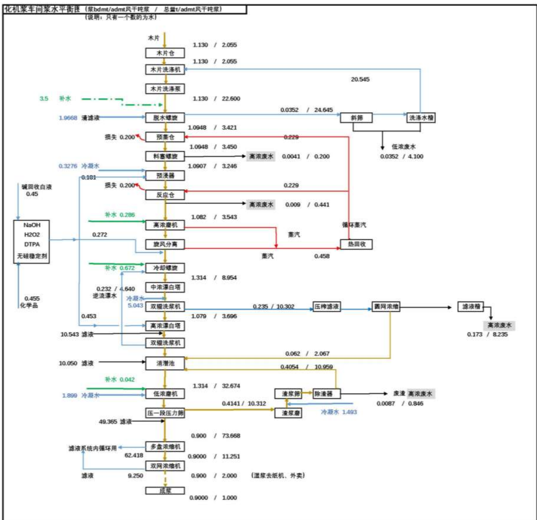
图3.2-13化机浆浆水平衡图 (t/t干浆)
