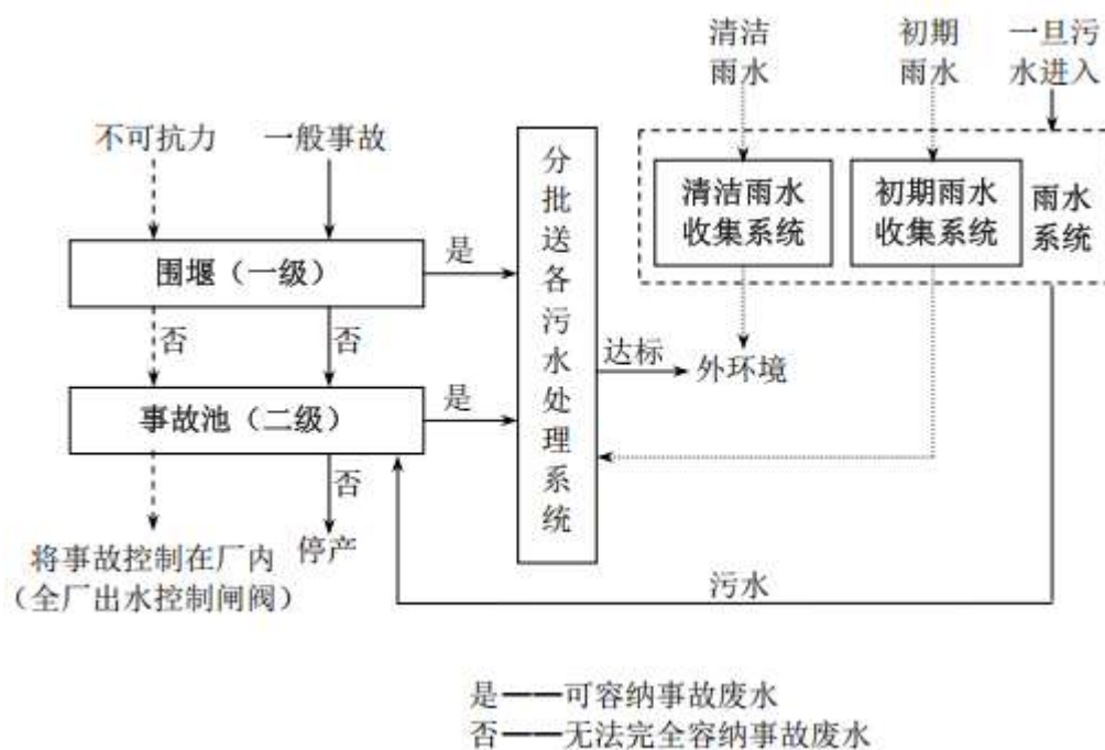
图7.10-3 厂区雨水风险防范措施示意图
