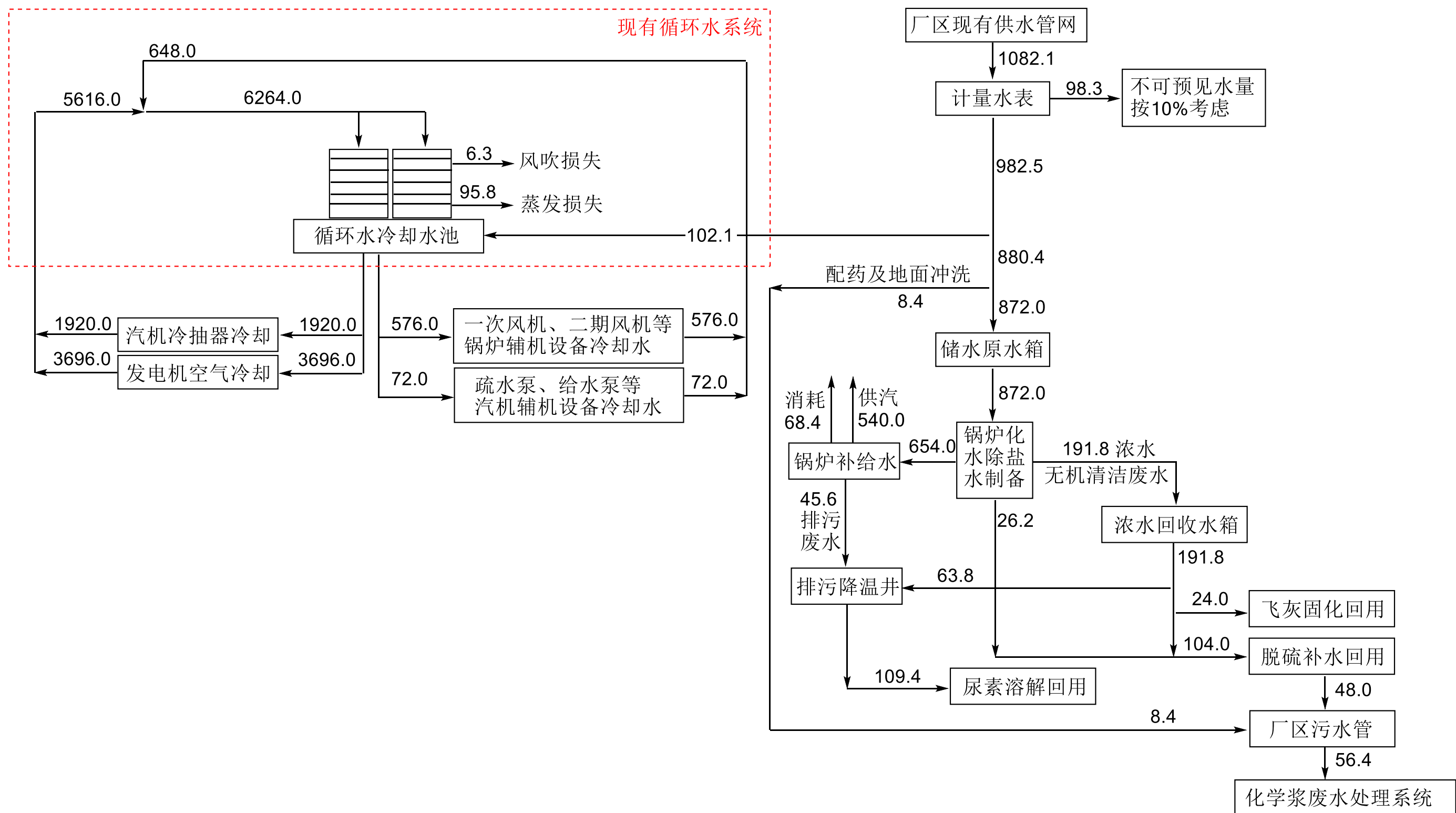
图3.2-23配套建设固废资源综合利用项目水平衡图（t/d）
