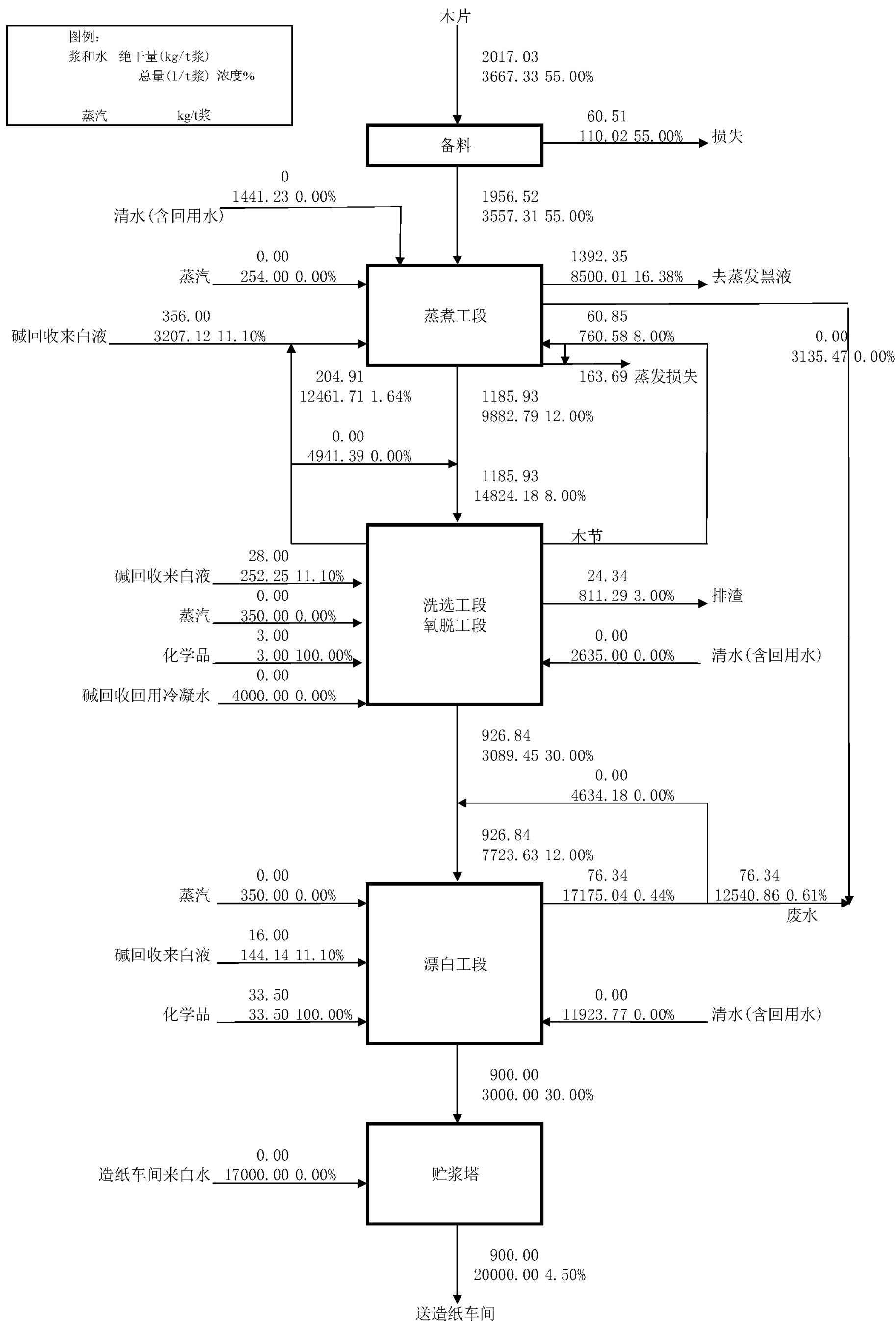
图3.2-16化学浆浆水平衡图 (t/t 干浆)
