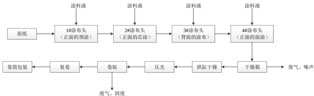
图2.3-3 涂布工艺流程图
