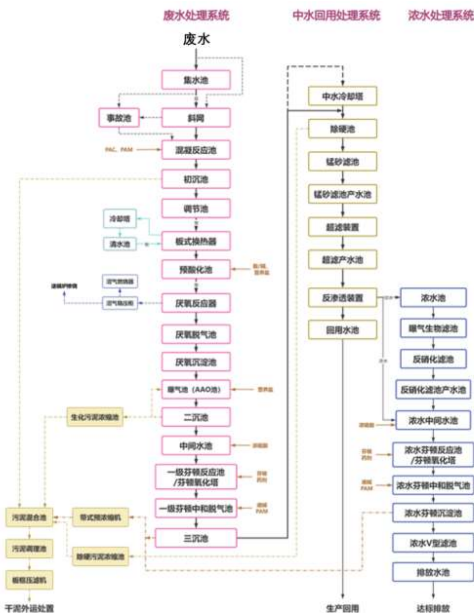
图8.2-3废水处理工艺流程图
