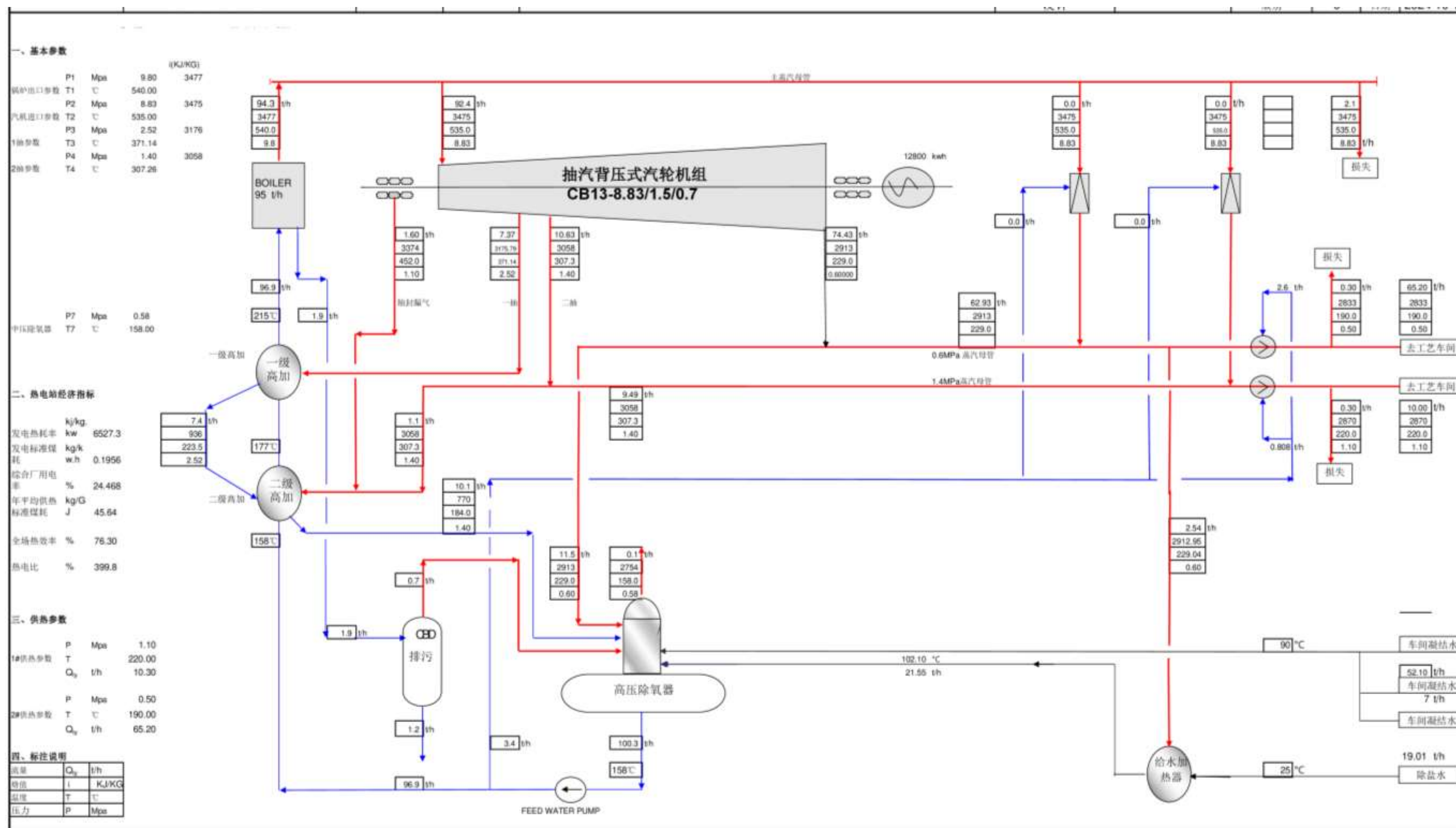
图3.2-22配套建设固废资源综合利用项目热平衡图
