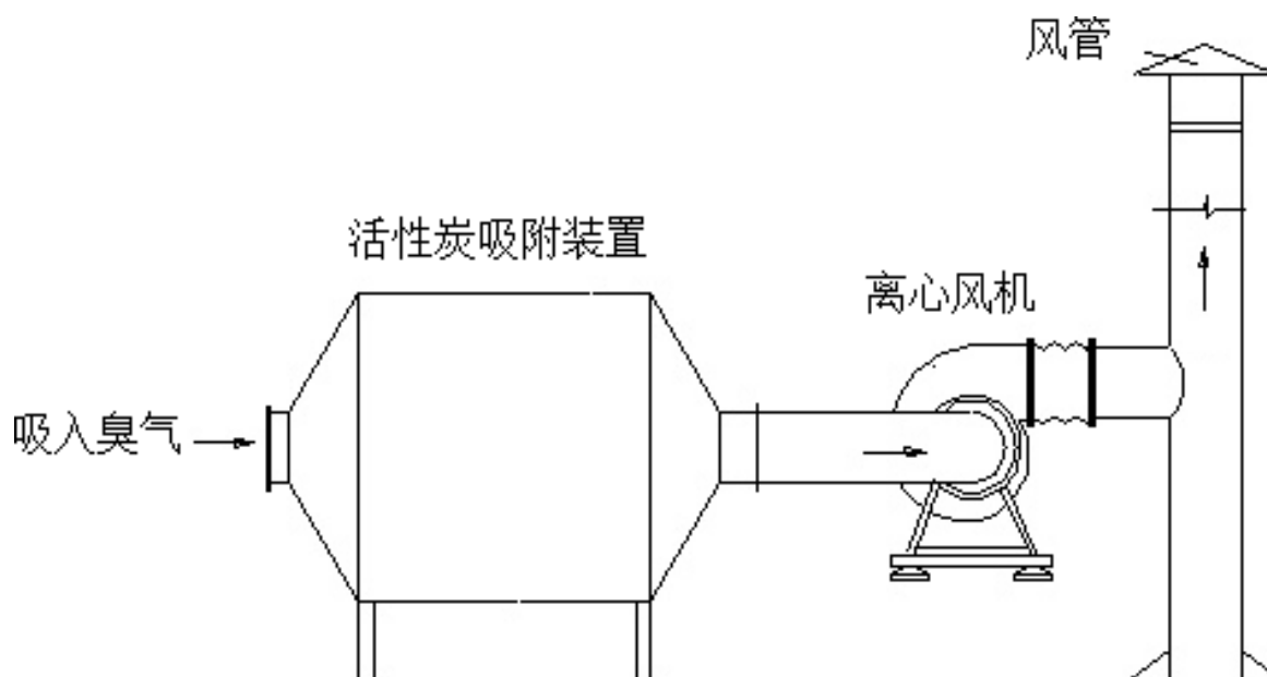
图8.2-2活性炭除臭装置系统流程图
