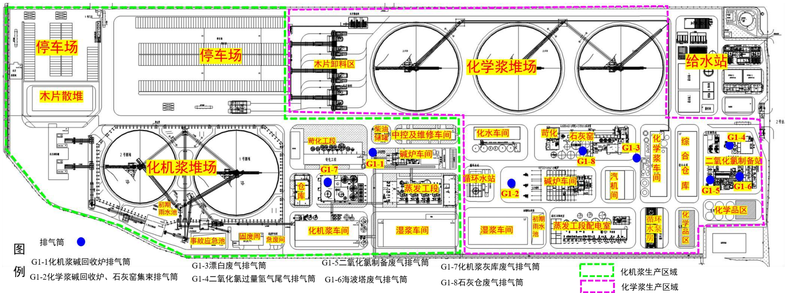
图3.1-1制浆生产区（地块一）平面布置图
