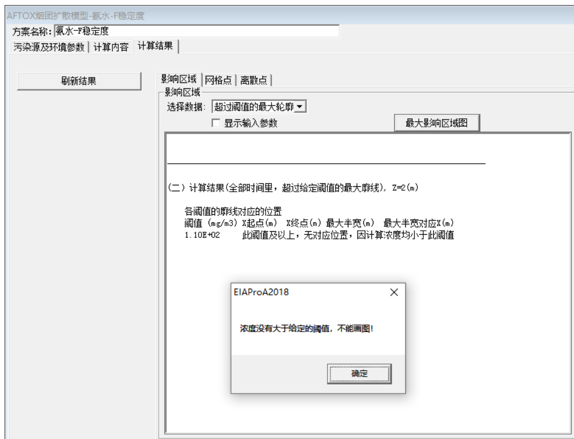
图7.7-12最常见气象条件下氨水储罐泄漏最大影响范围图
