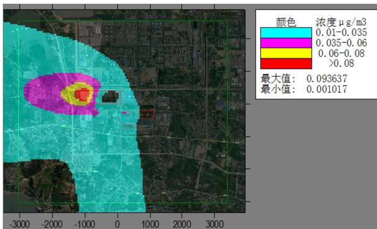
图6.1-12评价范围内最大年平均 \text{PM}_{10} 地面浓度增量空间分布
