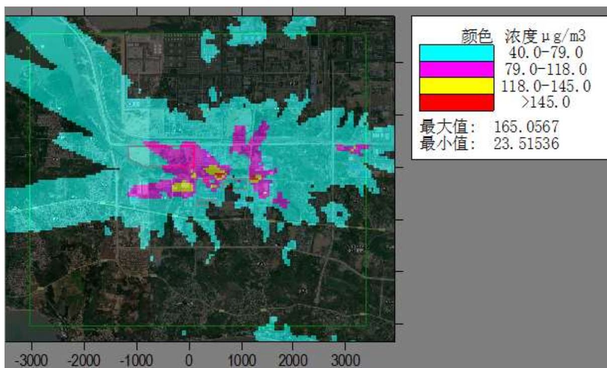
图6.1-45叠加区域源和背景浓度 \text{NH}_3 小时均浓度空间分布
