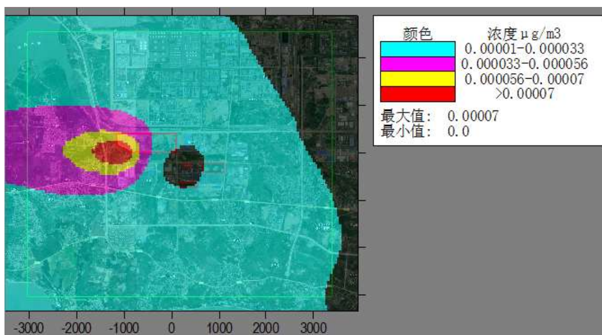
图6.1-28评价范围内最大年平均铅地面浓度增量空间分布
