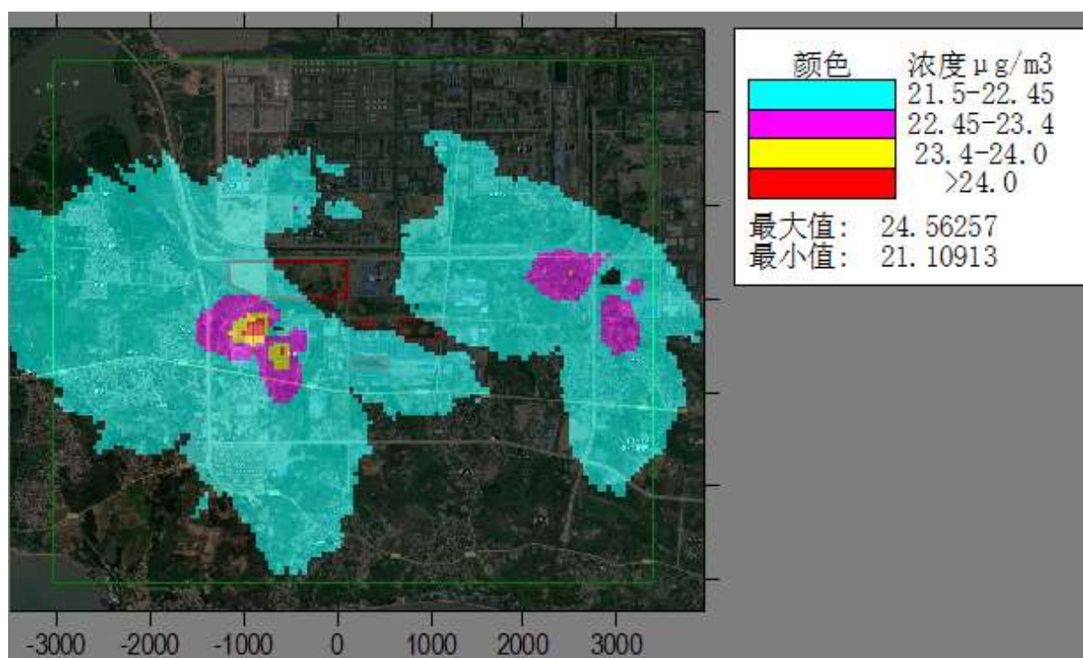
图6.1-31叠加区域源和背景浓度 98%保证率 \text{SO}_2 日平均浓度空间分布
