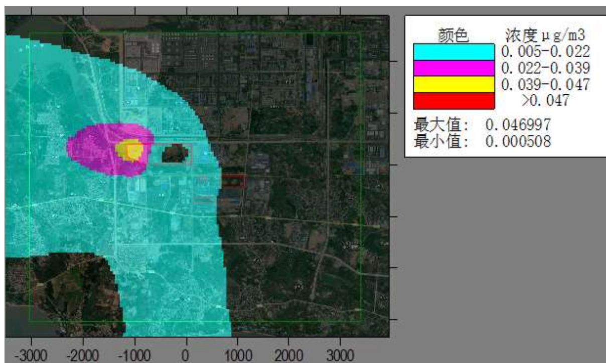
图6.1-14评价范围内最大年平均 \text{PM}_{2.5} 地面浓度增量空间分布
