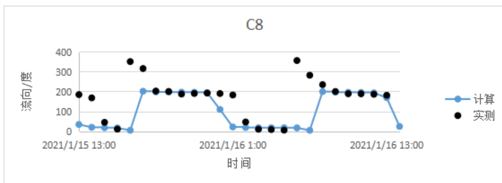
图6.2-13C8 流向、流速验证曲线
