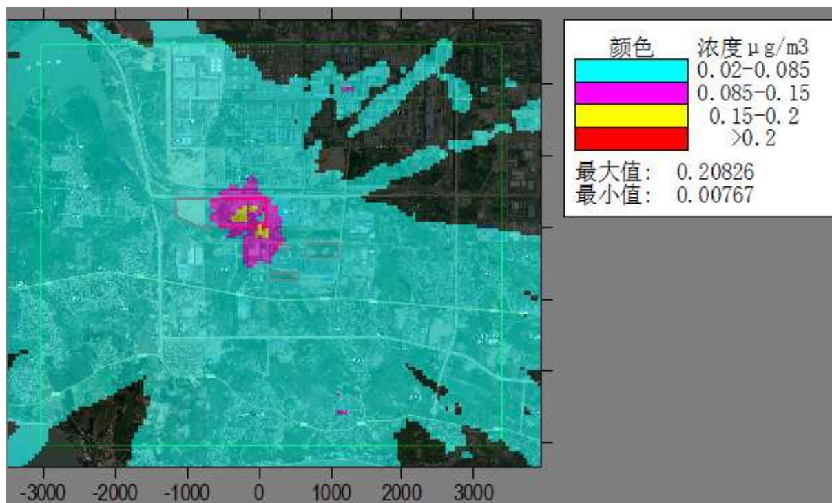
图6.1-21评价范围内最大日平均 HCl 地面浓度增量空间分布
