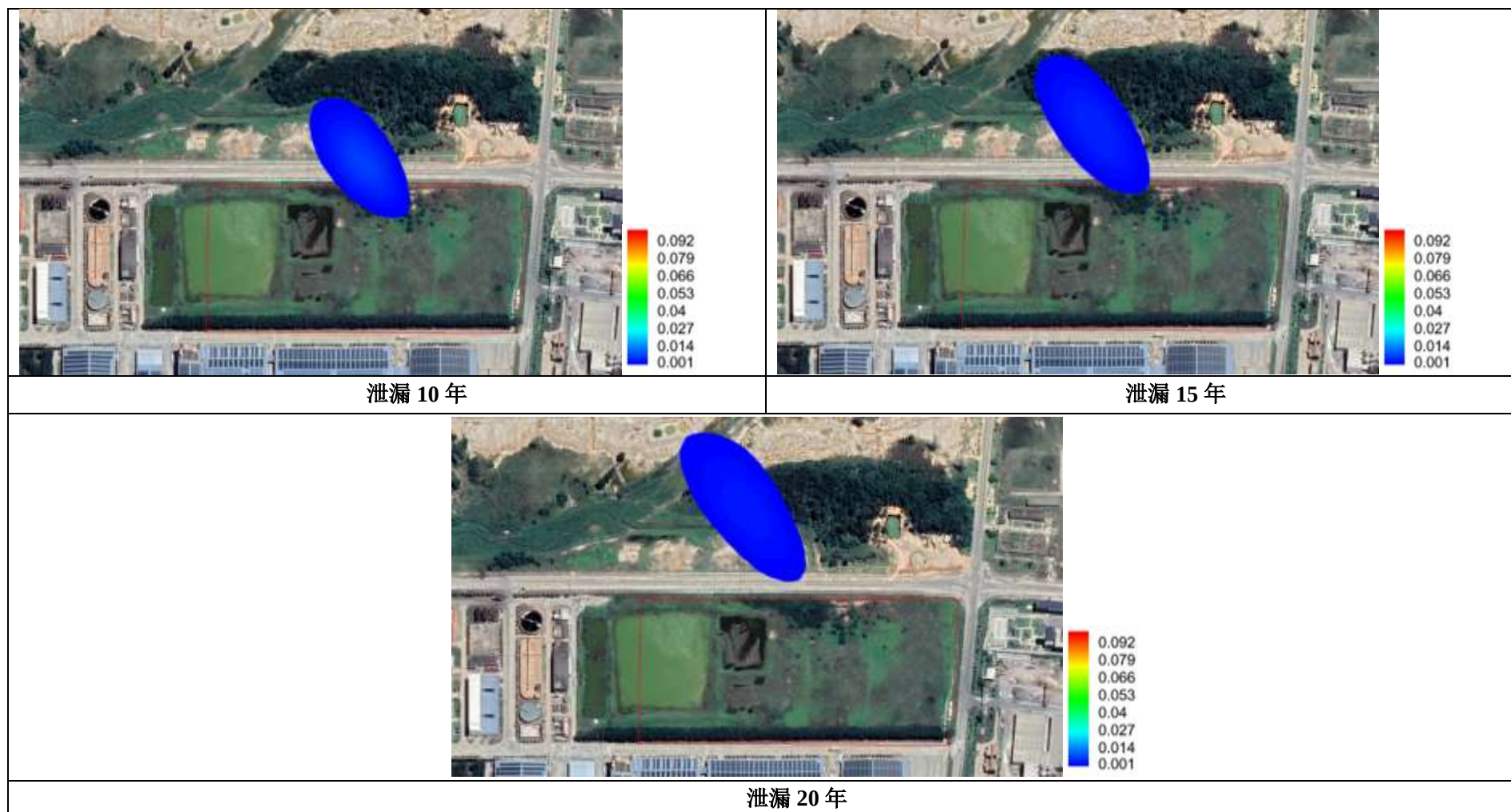
图6.3-11化学浆水处理系统调节池泄漏 COD 预测结果图
