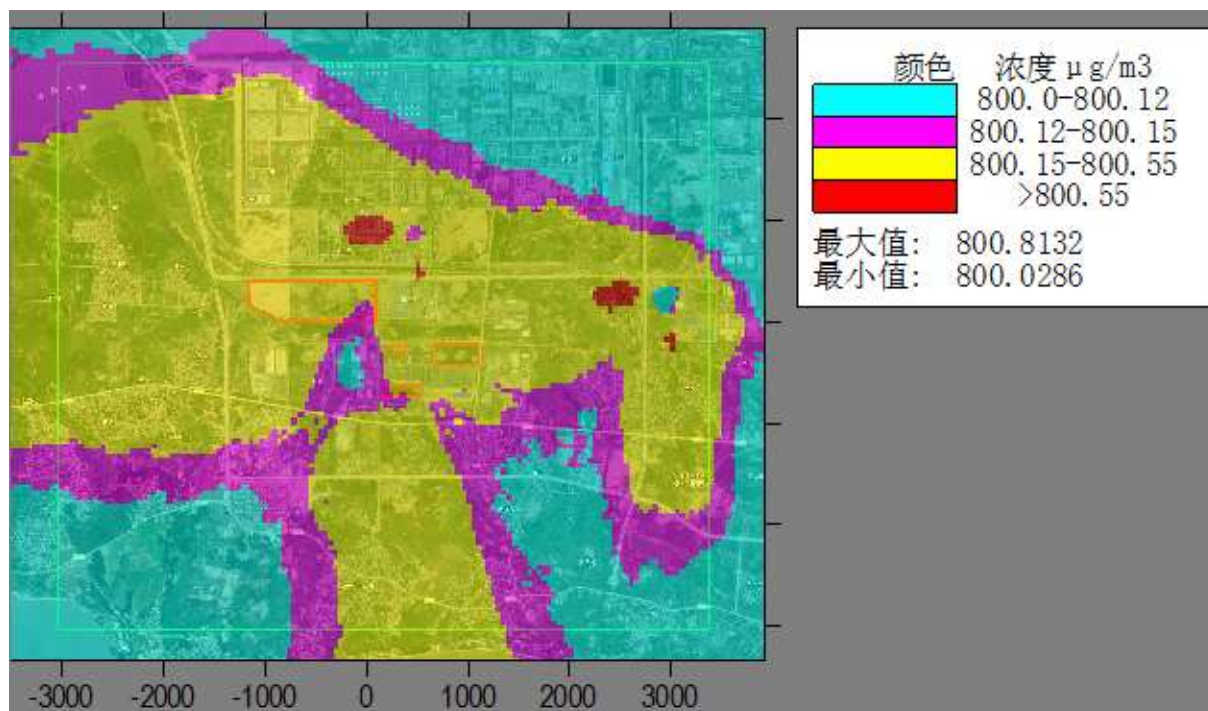
图6.1-39叠加区域源和背景浓度 95%保证率 CO 日平均浓度空间分布
