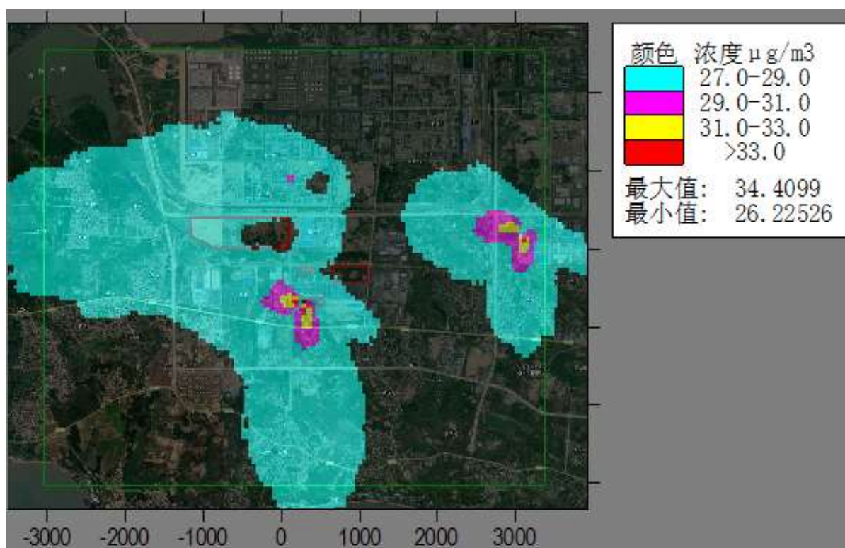
图6.1-33叠加区域源和背景浓度 98%保证率 \text{NO}_x 日平均浓度空间分布
