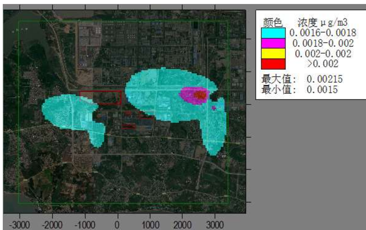
图6.1-49叠加区域源和背景浓度 Hg 年均浓度空间分布
