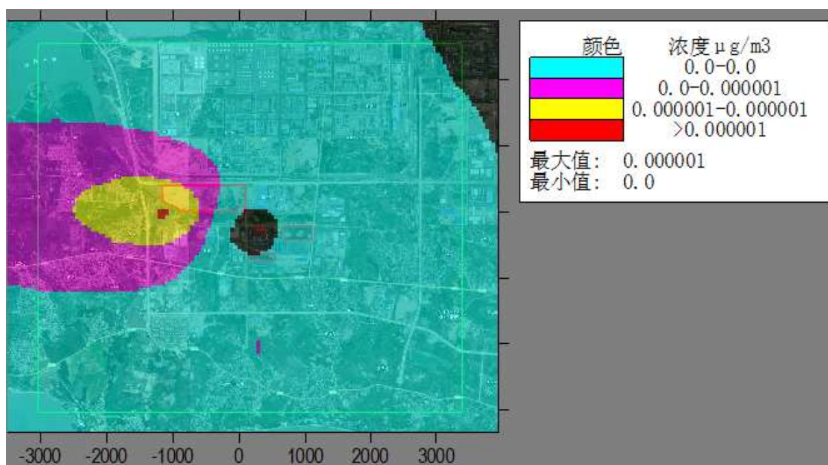
图6.1-54叠加区域源和背景浓度二噁英年均浓度空间分布
