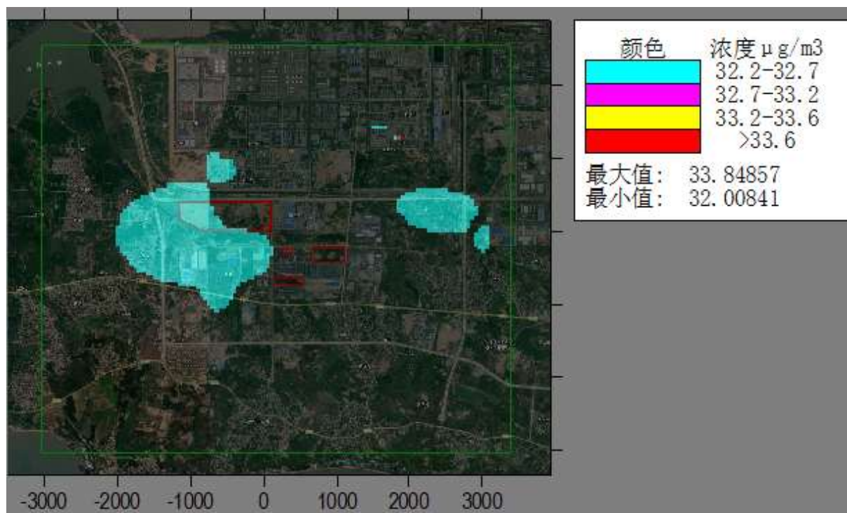
图6.1-36叠加区域源和背景浓度 \text{PM}_{10} 年均浓度空间分布
