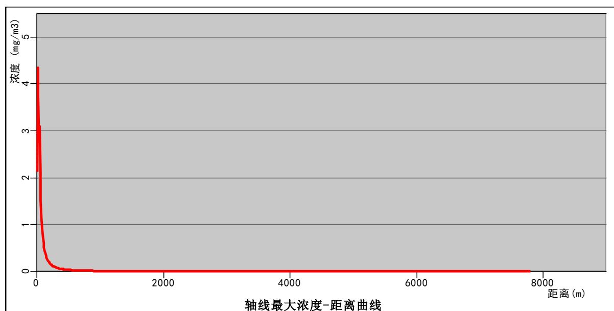
图7.7-1最常见气象条件下地块一盐酸储罐泄漏轴线最大浓度—距离曲线图
