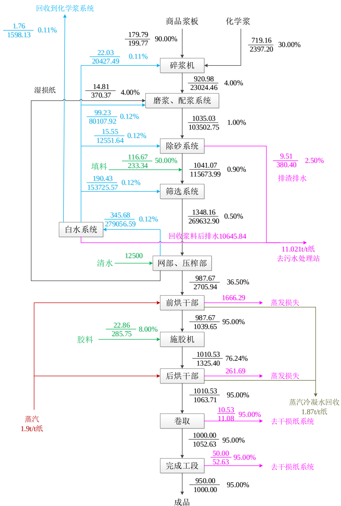
图3.2-20特种纸浆水平衡图(t 浆/t)
