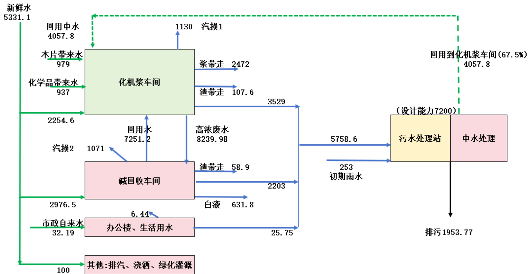
图3.2-15化机浆车间水平衡图 (t/d)
