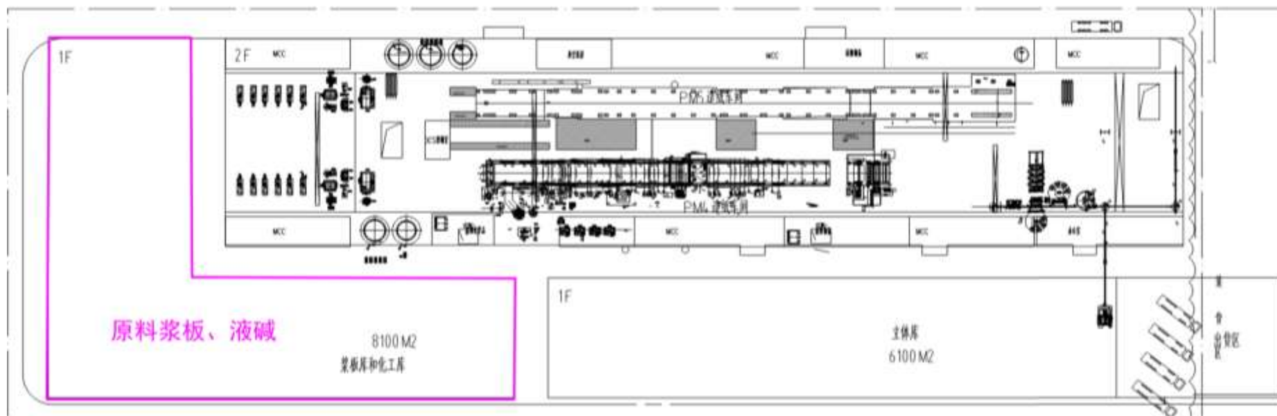
图7.5-4厂区危险单元分布图（地块四）
