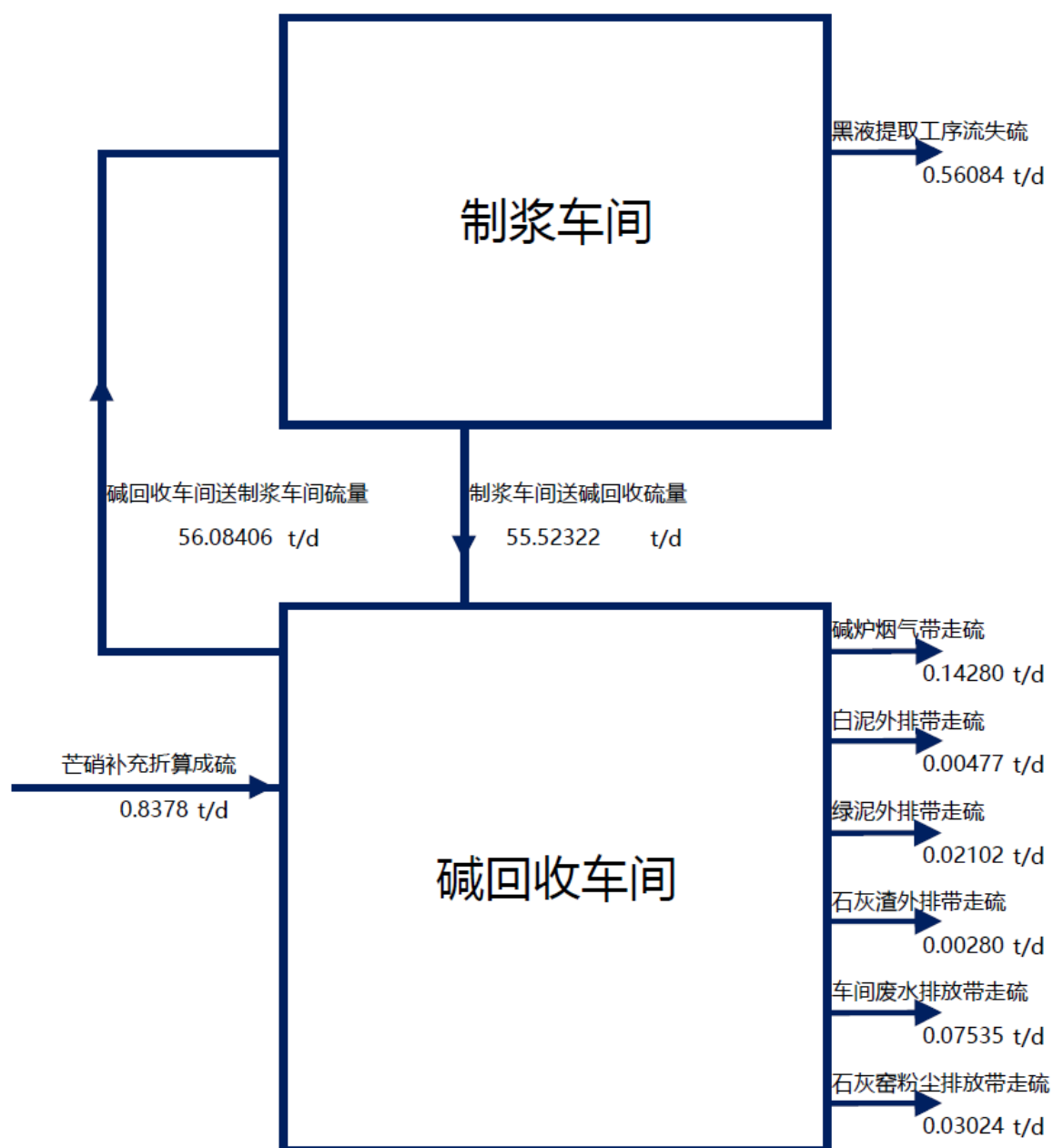
图3.2-18化学浆硫平衡（以 S 计，t/d）
