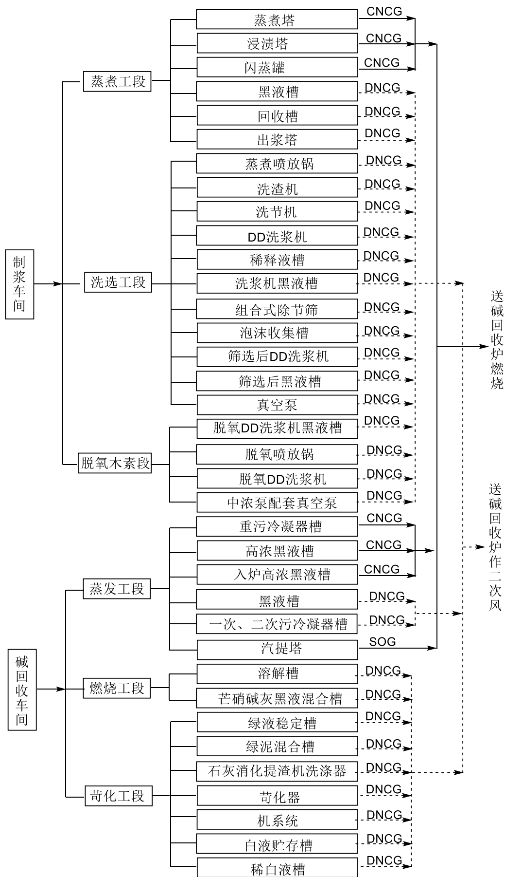
图3.2-8臭气收集处理示意图
