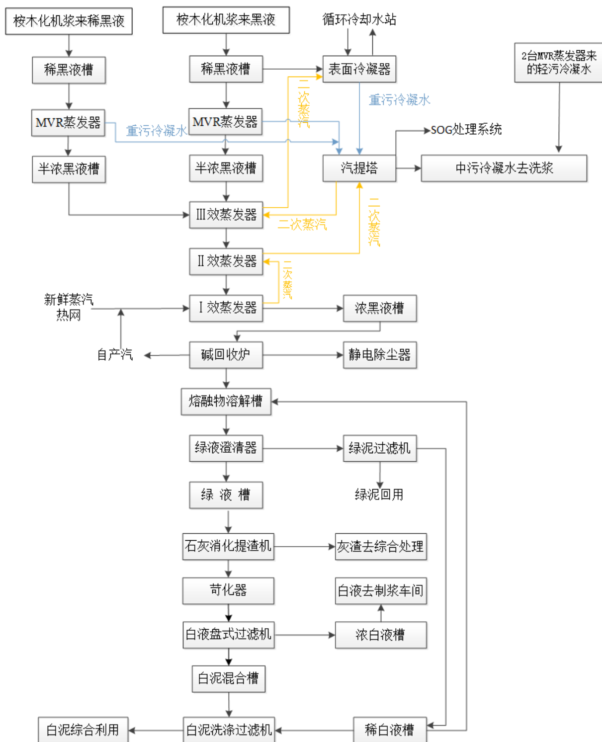
图3.2-4碱回收车间工艺流程及产污节点图
