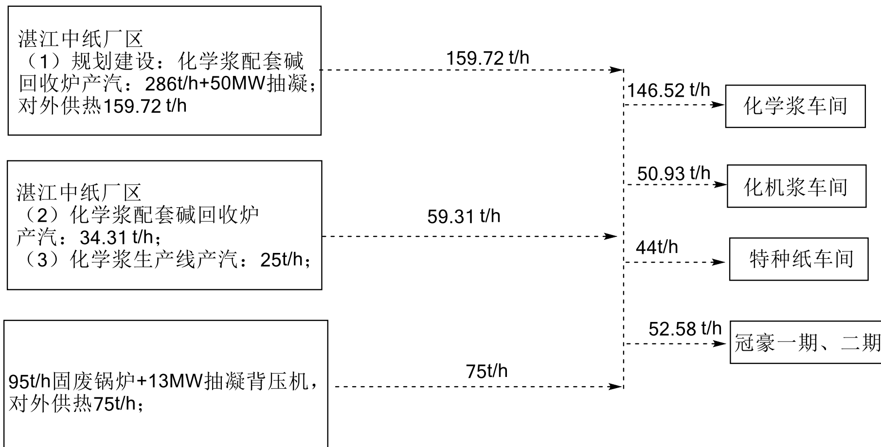
图3.2-26全厂蒸汽平衡 (t/h)
