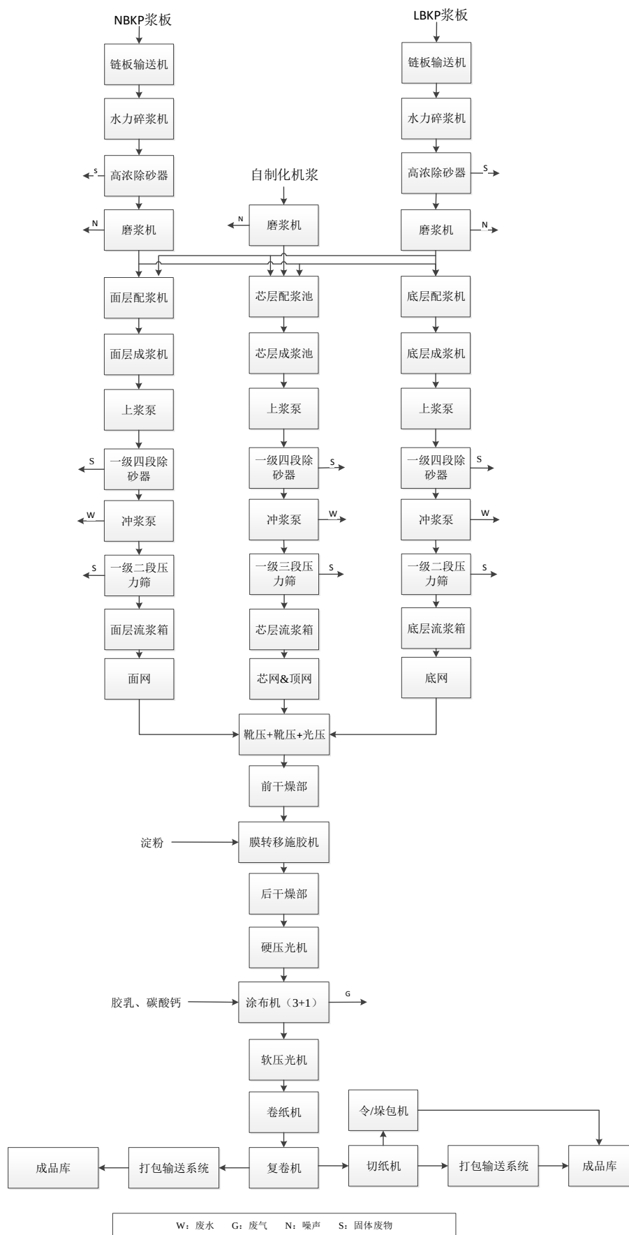
图2.3-4 涂布白卡纸生产工艺流程图及产污环节
