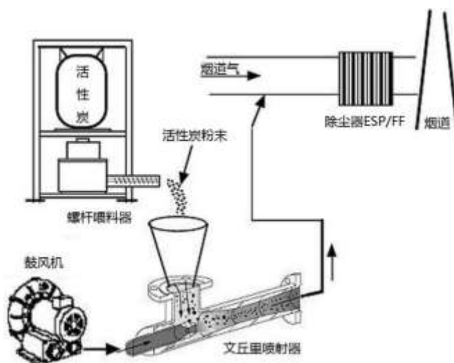
图8.2-1活性炭喷射系统
