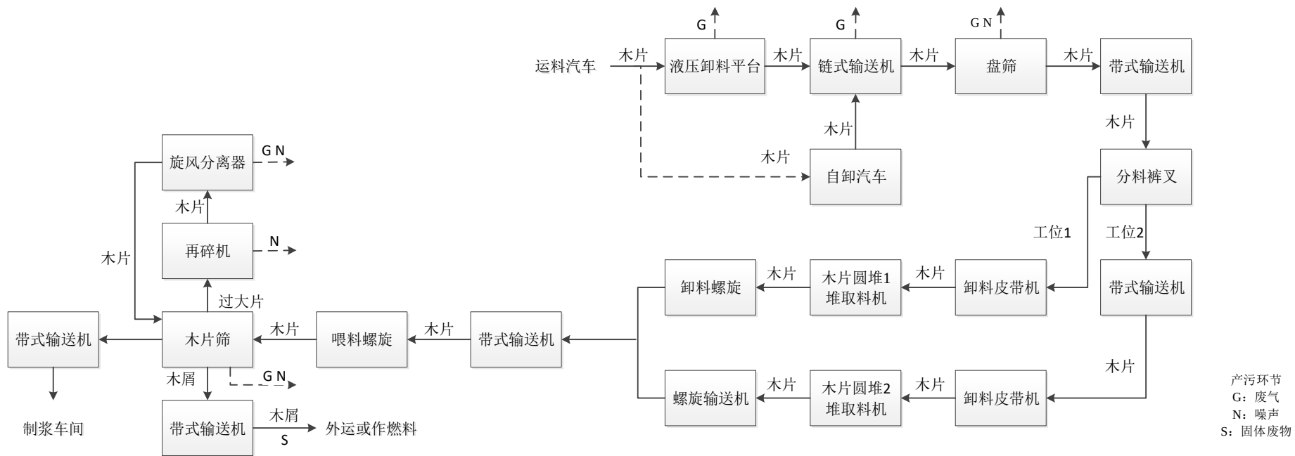
图3.2-1备料工段工艺流程及主要产污节点图
