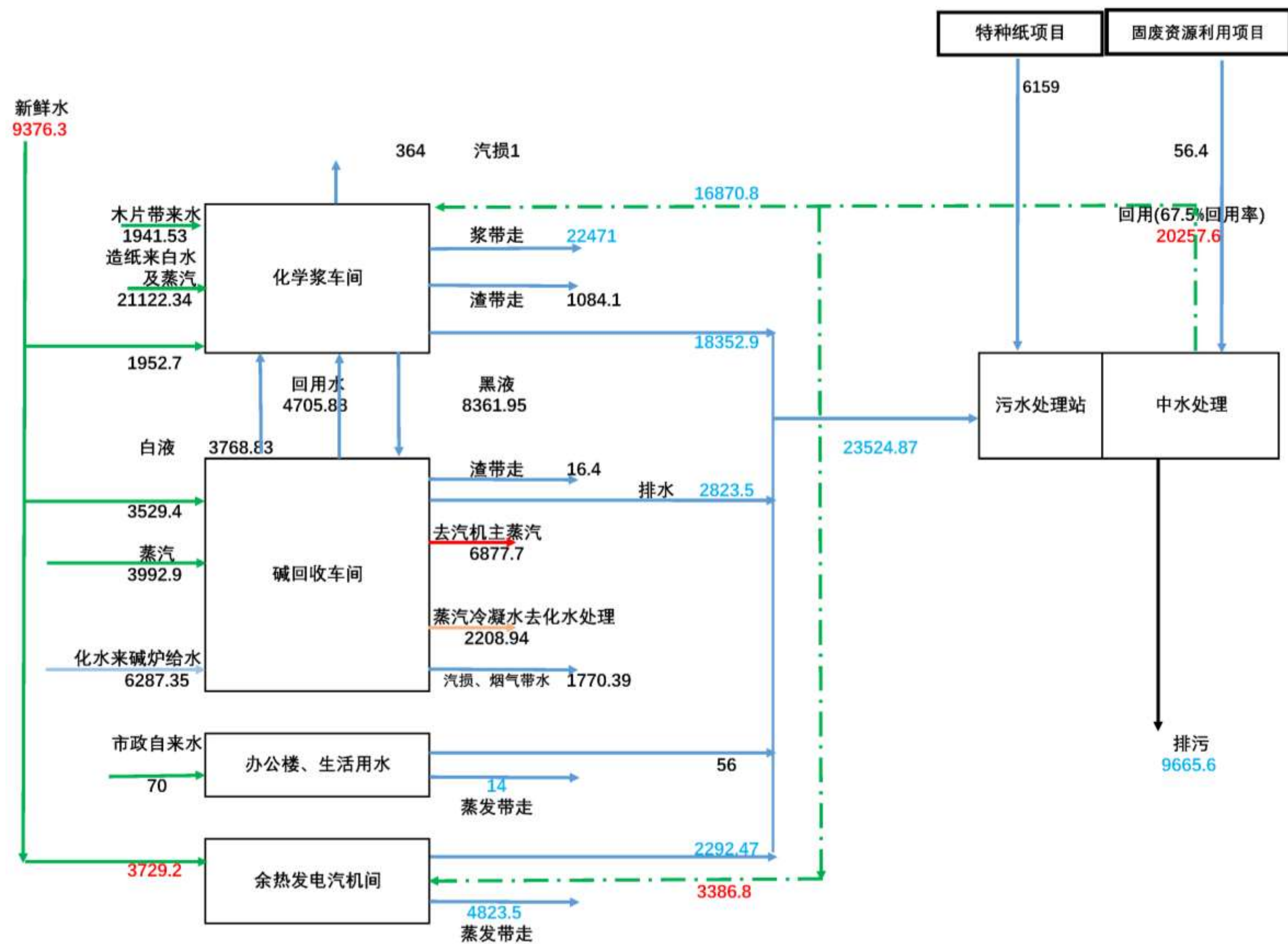
图3.2-24化学浆废水处理系统（含特种纸、配套建设固废资源综合利用项目废水）水平衡图（t/d）
