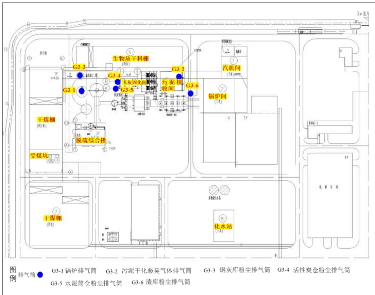
图3.1-3配套建设固废资源综合利用项目平面布置图
