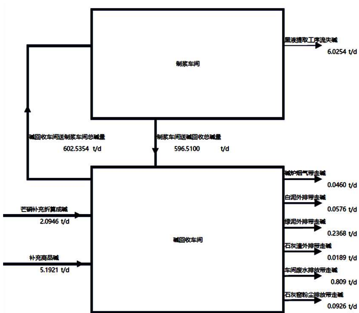
图3.2-17化学浆碱平衡 (t/d, 以 100%NaOH 计)
