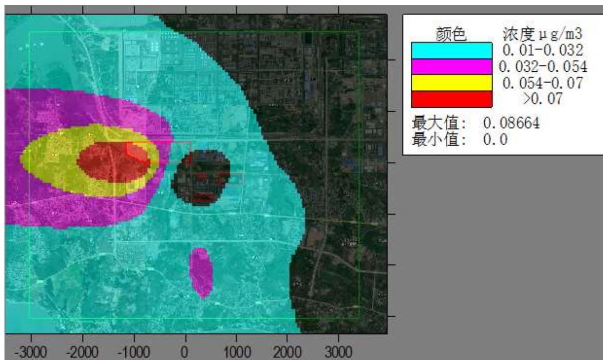
图6.1-17评价范围内最大年平均 CO 地面浓度增量空间分布
