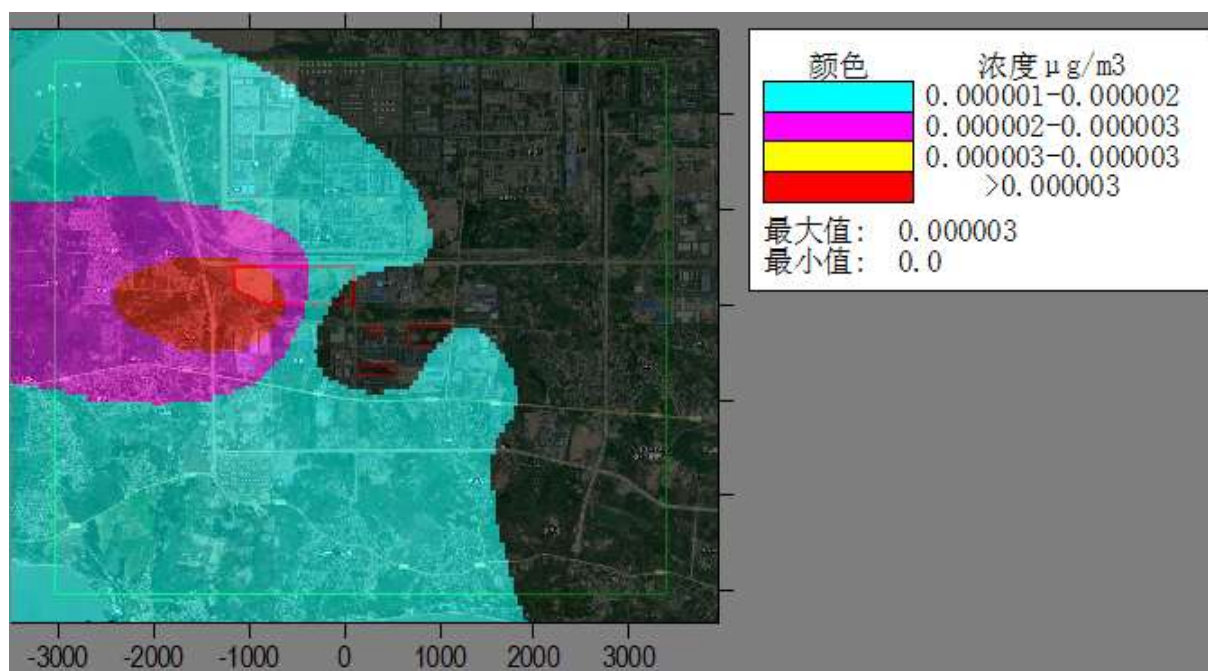
图6.1-26评价范围内最大年平均汞地面浓度增量空间分布
