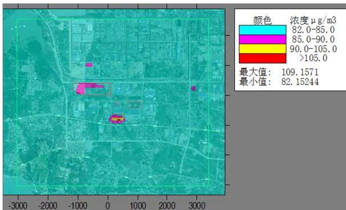
图6.1-48叠加区域源和背景浓度 TSP 年均浓度空间分布
