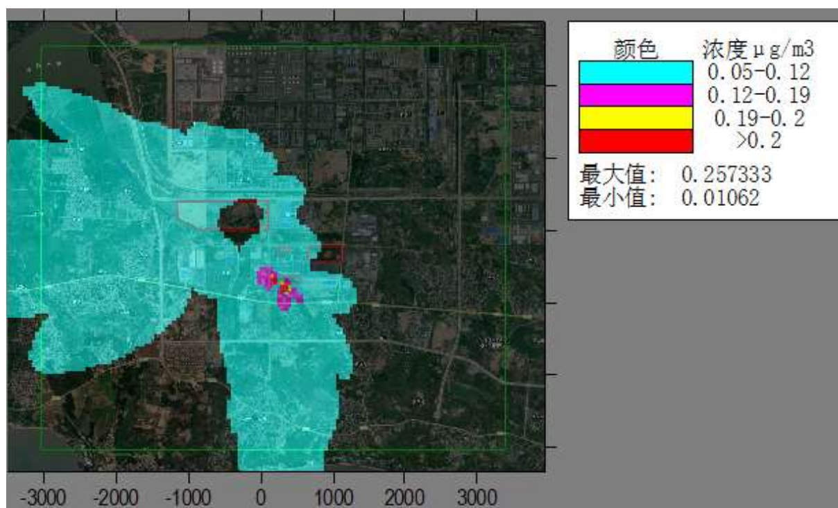
图6.1-6评价范围内最大日平均SO 2 地面浓度增量空间分布
