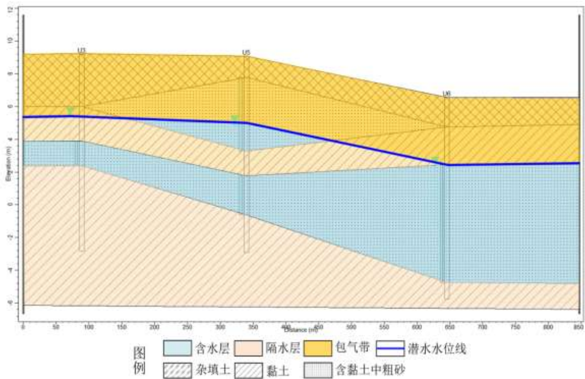
图6.3-2龙腾河以北地块水文地质剖面示意图
