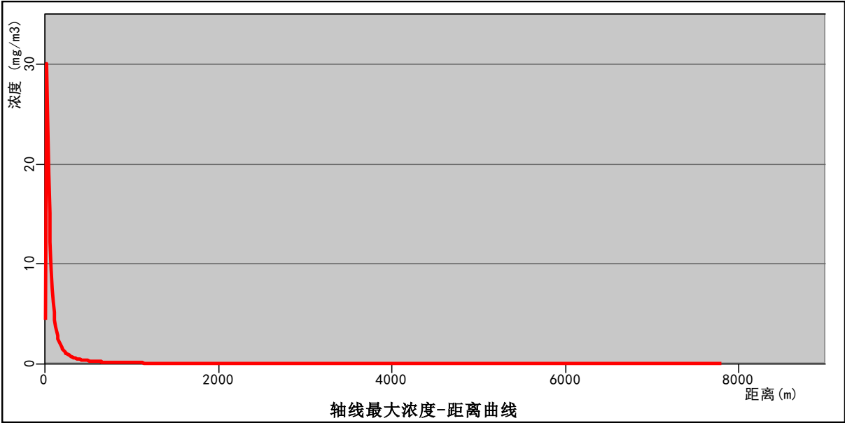
图7.7-9最常见气象条件下氨水储罐泄漏轴线最大浓度—距离曲线图
