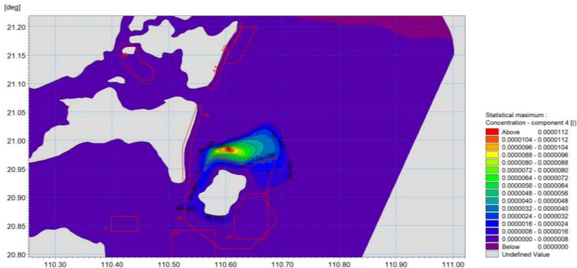
图6.2-19正常排放情况下总铬浓度增量最大值分布包络线图
