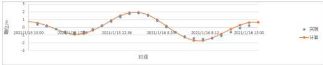
图6.2-5 T2 潮位验证曲线
