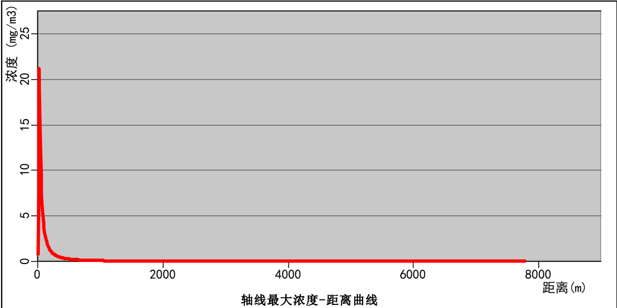
图7.7-7最不利气象条件下地块二盐酸储罐泄漏轴线最大浓度—距离曲线图
