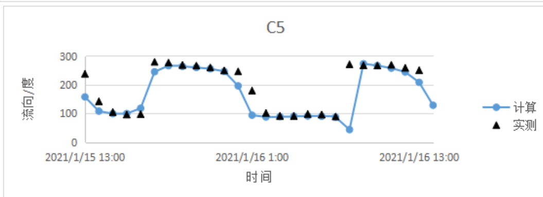
图6.2-10C5 潮流流向、流速验证曲线
