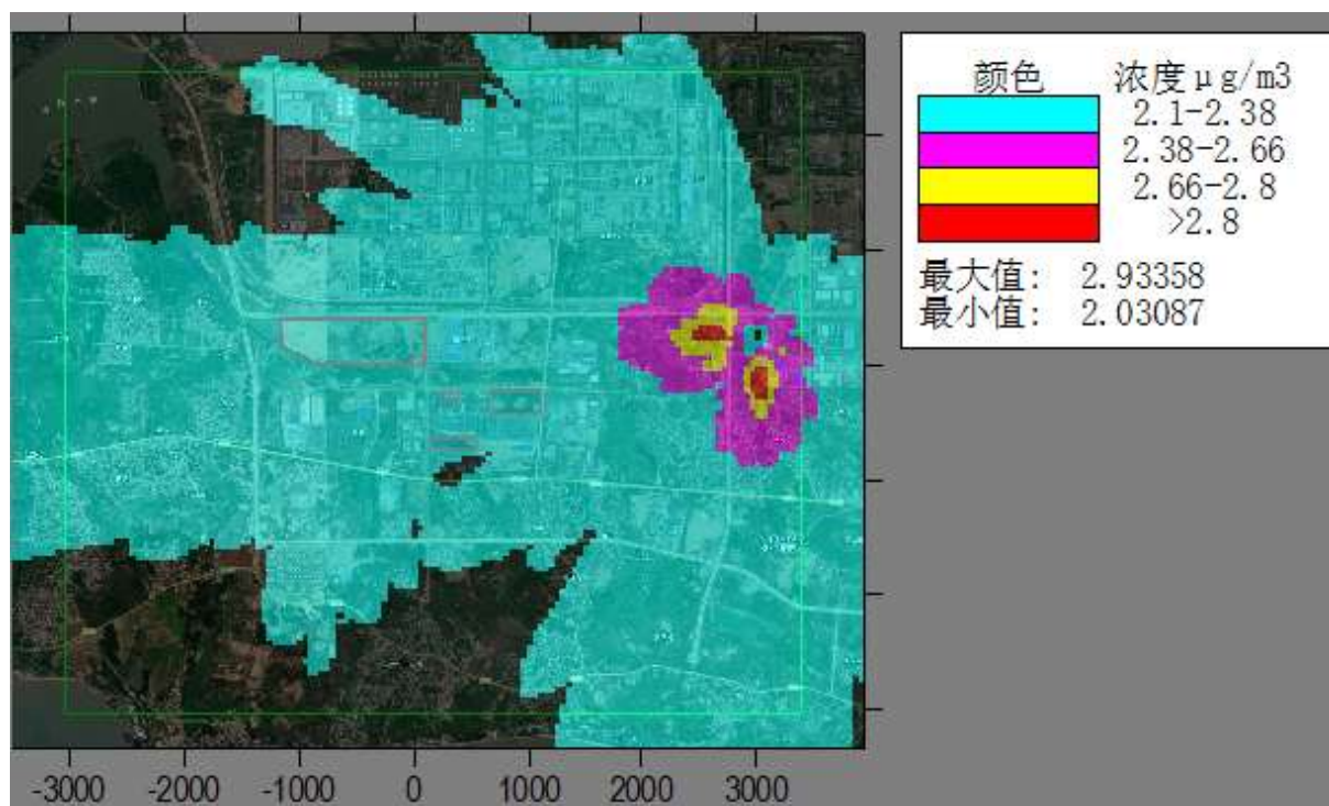
图6.1-44叠加区域源和背景浓度 HCl 日均浓度空间分布
