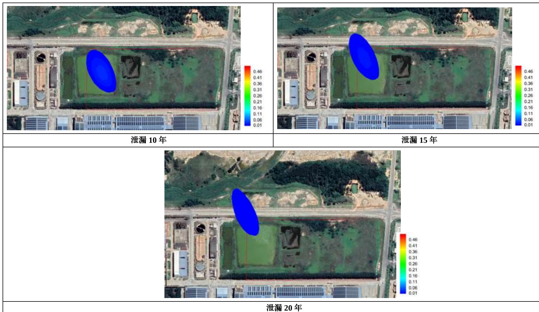
图6.3-10化机浆污水处理系统调节池泄漏 COD 预测结果图
