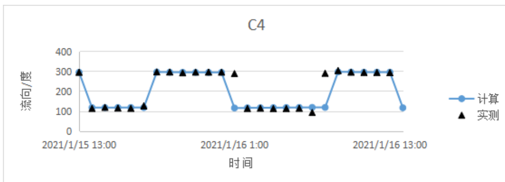
图6.2-9C4 潮流流向、流速验证曲线
