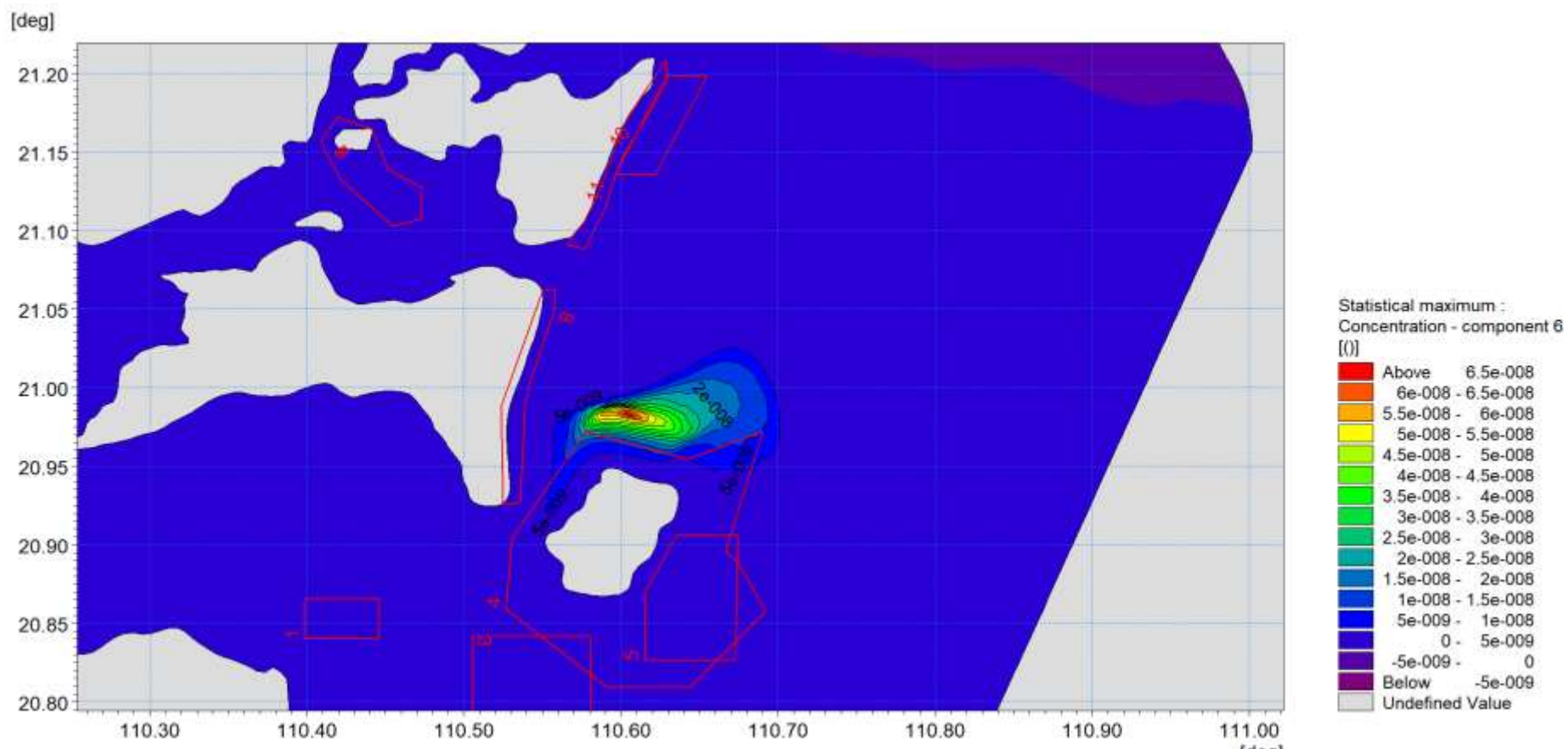
图6.2-27事故排放情况下二噁英浓度增量最大值分布包络线图
