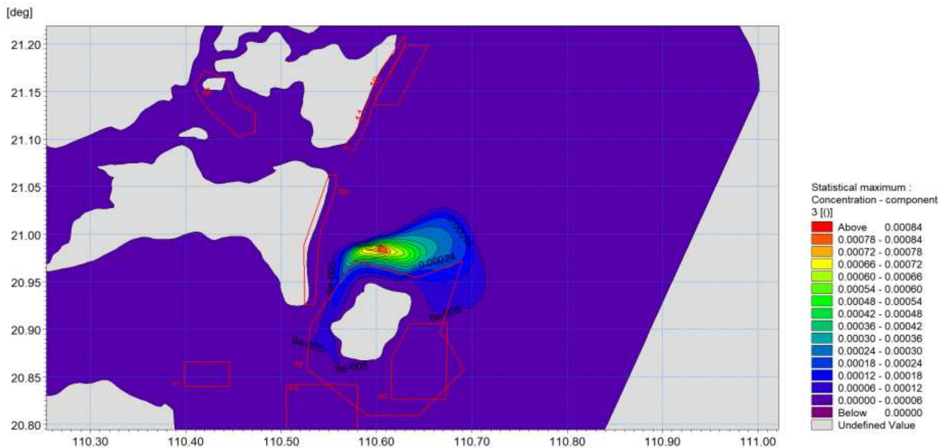
图6.2-18正常排放情况下活性磷酸盐浓度增量最大值分布包络线图
