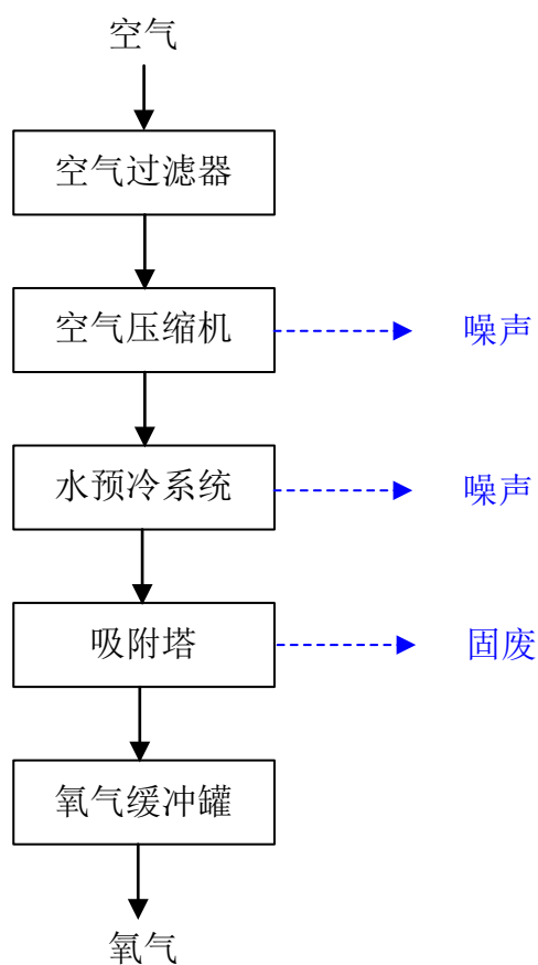
图3.2-6制氧站工艺流程图
