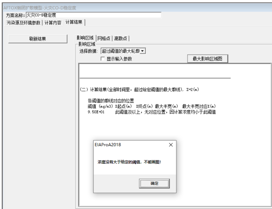
图7.7-18最常见条件下柴油储罐泄漏引发火灾产生 CO 最大影响范围图
