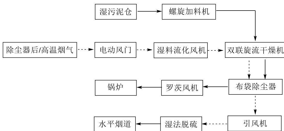
图3.2-12污泥干化系统工艺流程图
