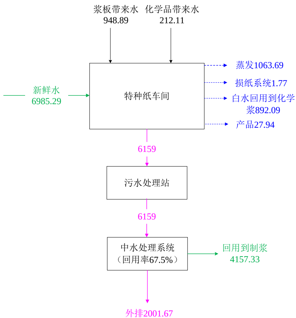
图3.2-21特种纸水平衡图 (t/d)
