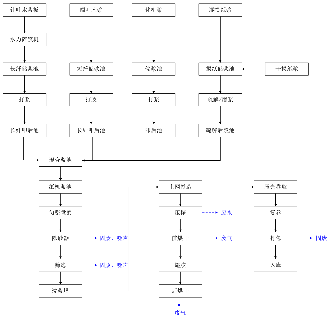
图3.2-10特种纸生产工艺流程图
