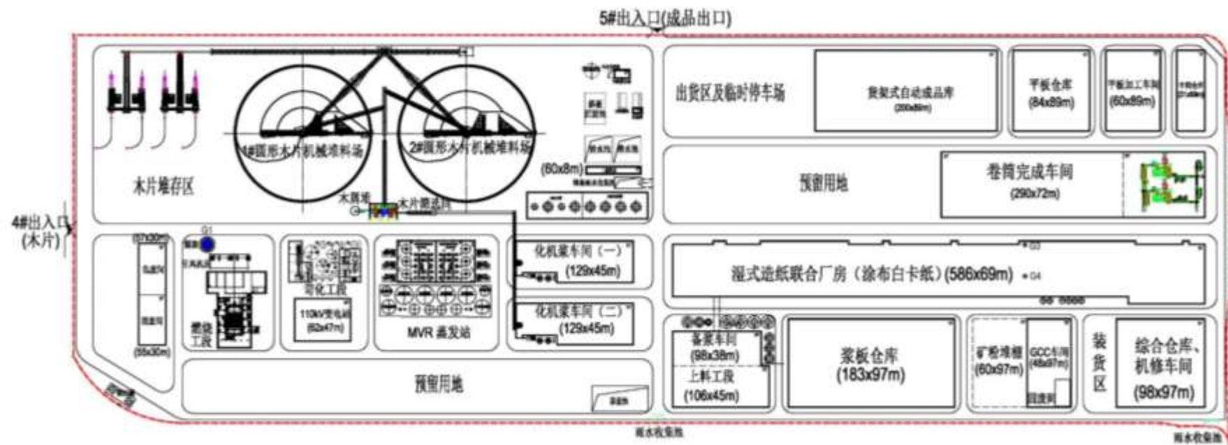
图2.2-2原地块一（制浆、造纸）平面布置示意图
