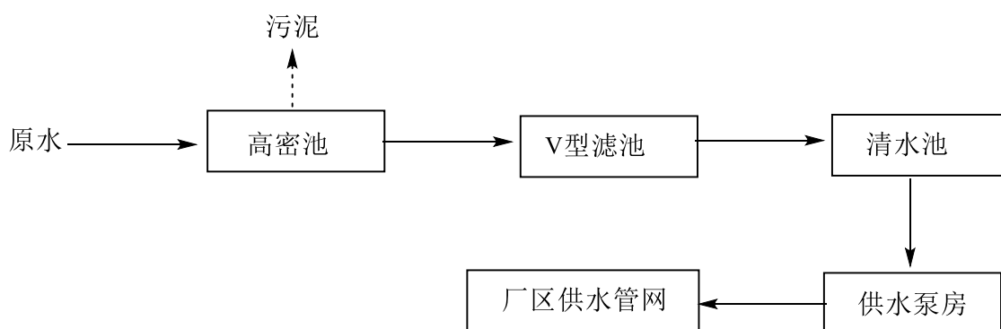
图3.1-5给水站工艺流程图
