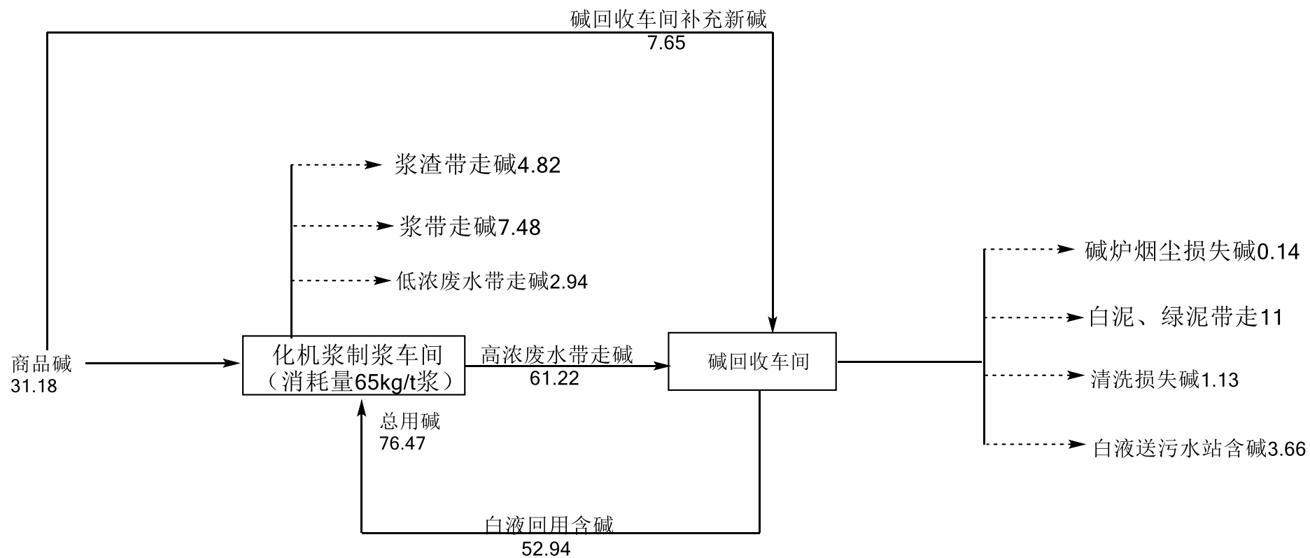
图3.2-14化机浆碱平衡(t/d, 以 100%NaOH 计)
