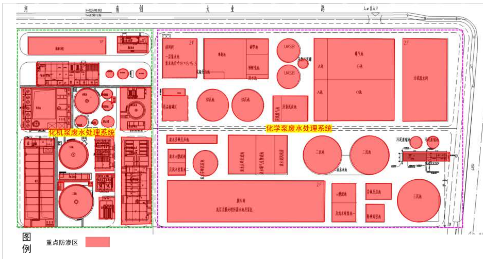
图8.2-5地块二地下水分区防渗图
