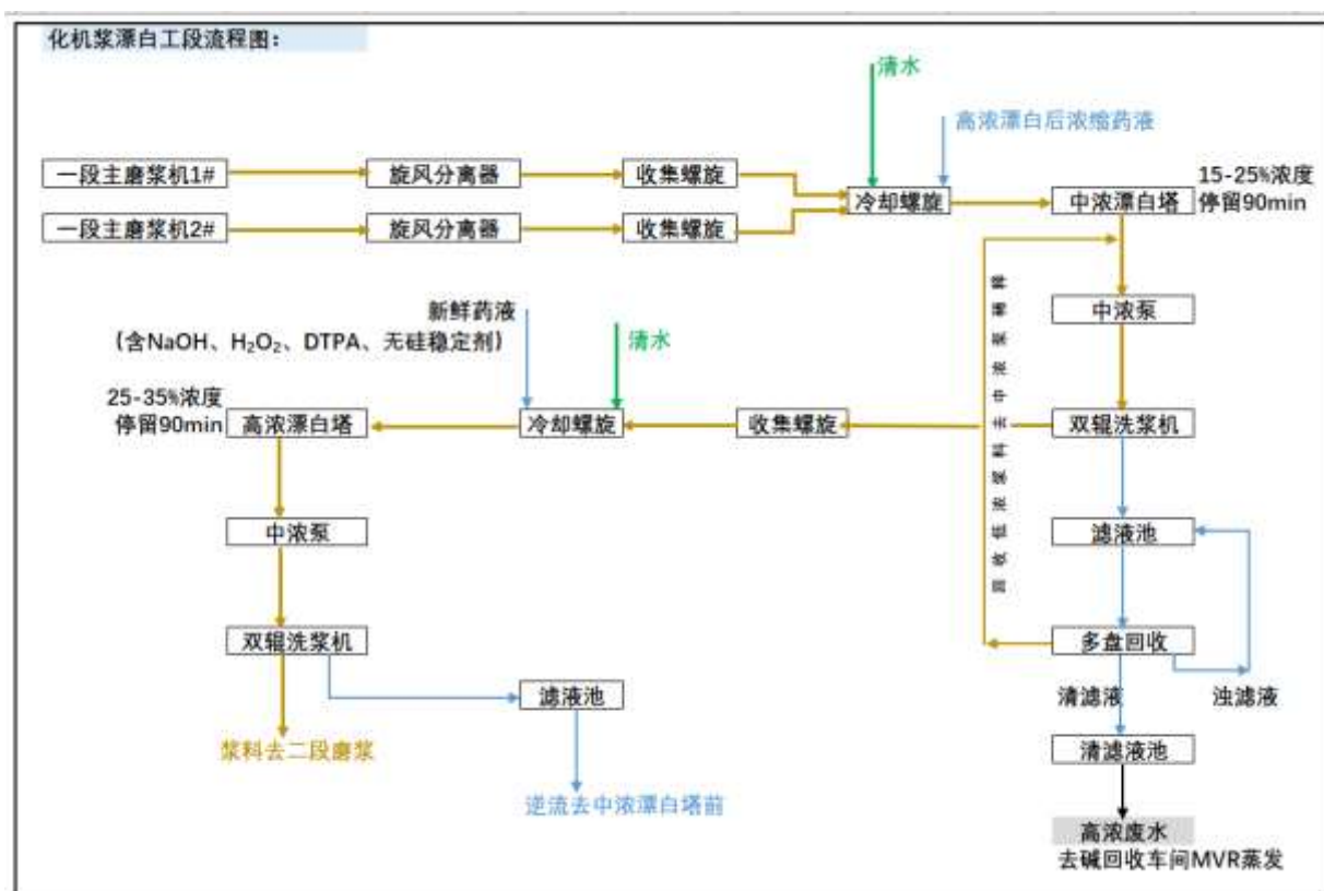
图3.2-3化机浆漂白工艺流程图
