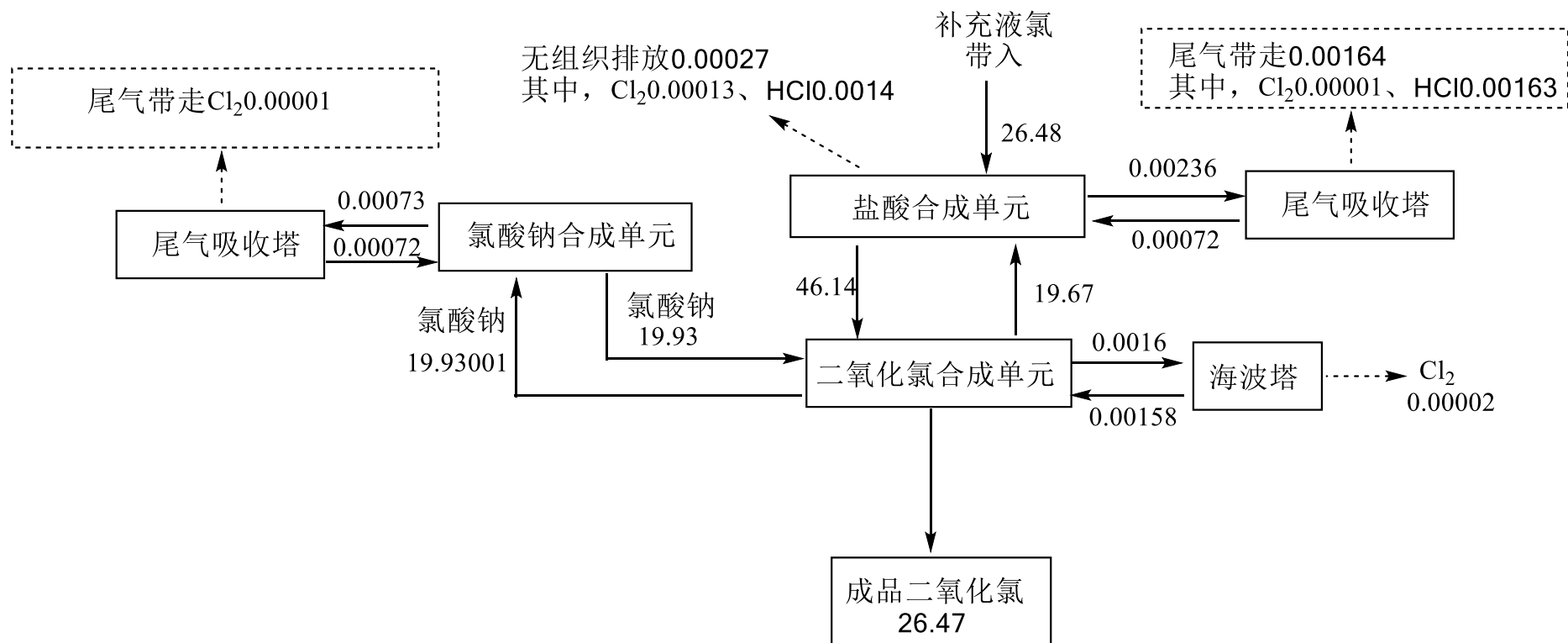
图3.2-19二氧化氯平衡图 (t/d)
