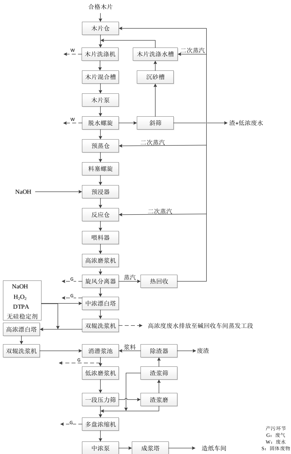
图3.2-2化机浆生产线工艺流程及产污节点图
