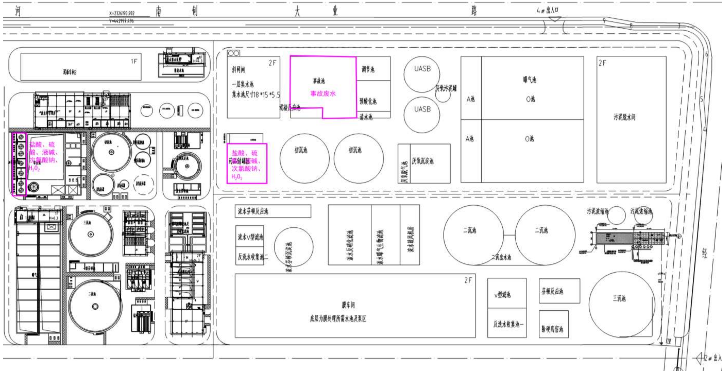
图7.5-2厂区危险单元分布图（地块二）
