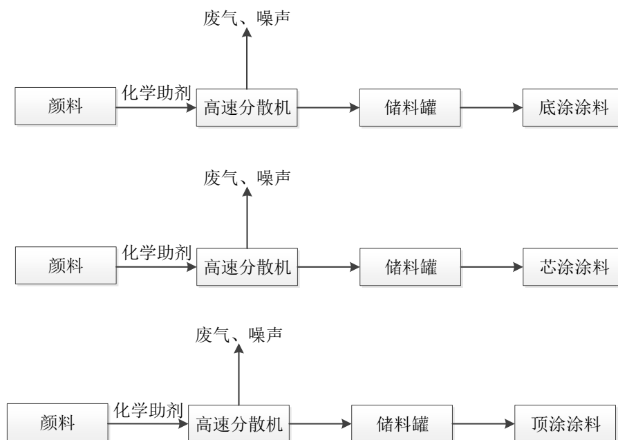
图2.3-2 涂料制备工艺流程图
