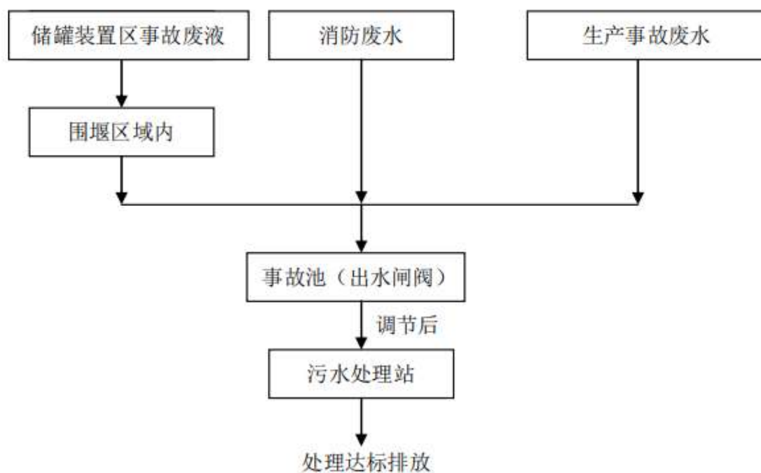
图7.10-1事故废水收集系统
